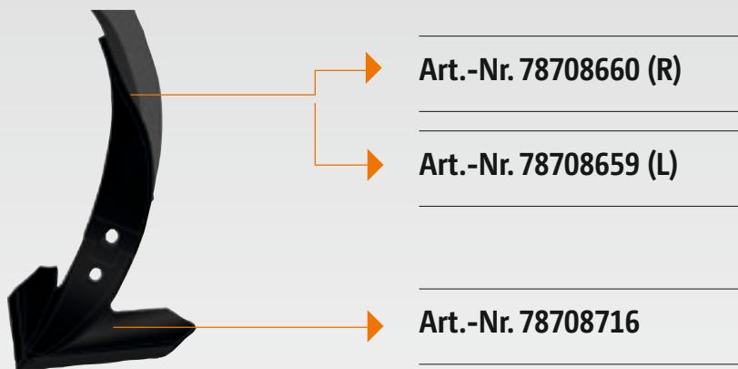
C-Mix 2 Gänsefußschar 320 mm mit C-Mix 2 Leitblech 100 mm C-Mix 2 duckfoot coulter 320 mm with 100 mm C-Mix 2 deflector guide
