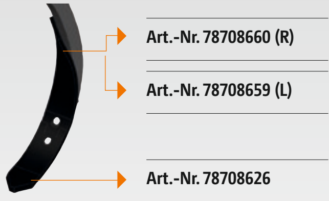
100 mm Scharspitze mit Leitblech 100 mm coulters with guide plate
